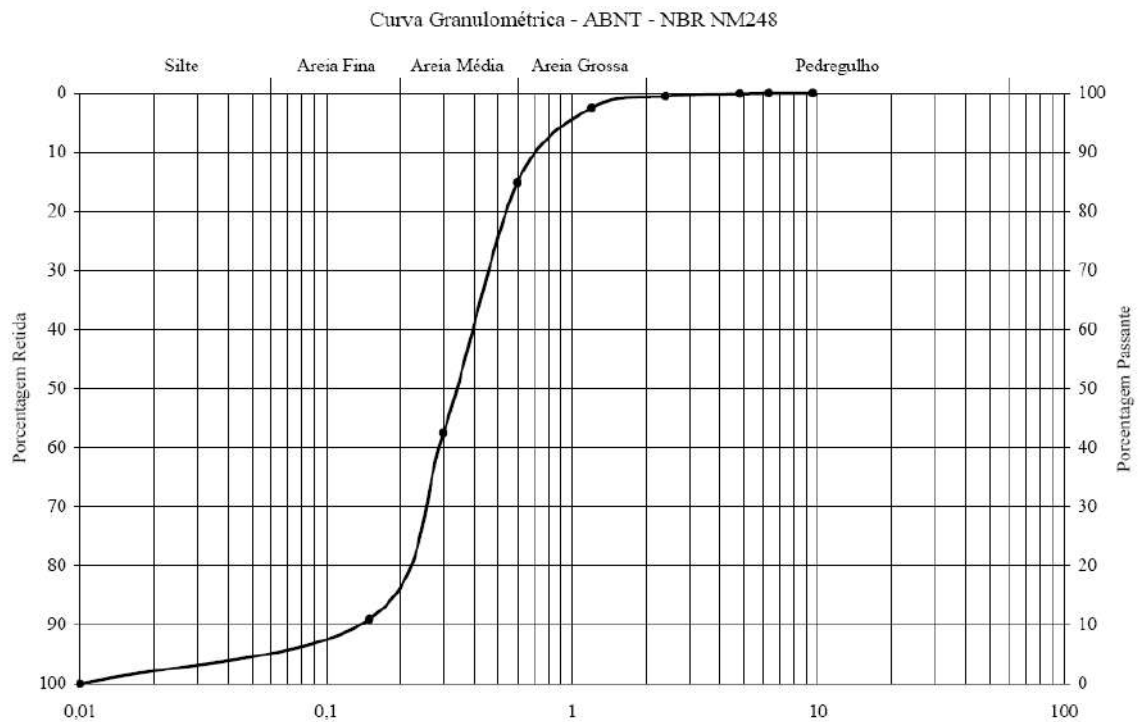
Figura 7 – Curva Granulométrica
