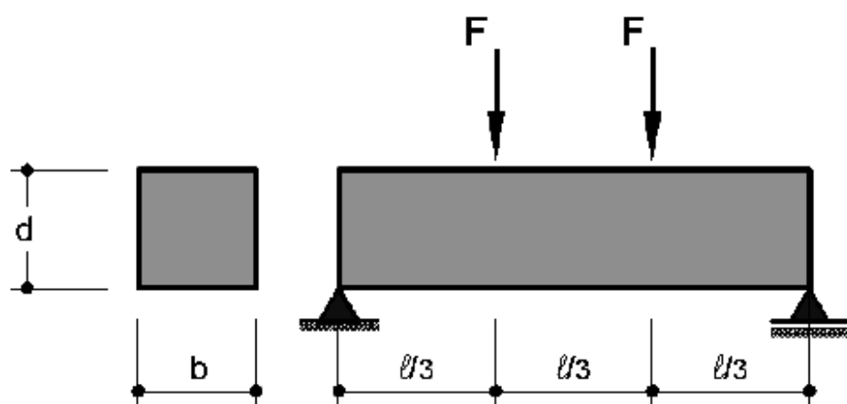
Figura 5.7 – Ensaio de tração na flexão
